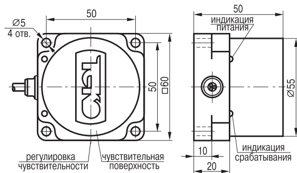
Габаритный чертёж
